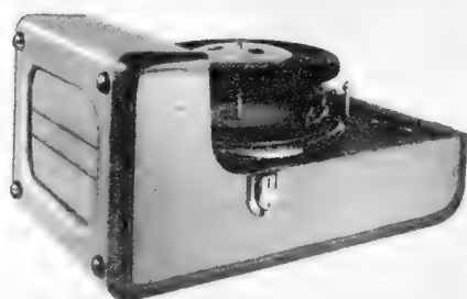
Bild 8. Phono-Verstärkerkoffer mit Plattenwechsler (Saemann)
