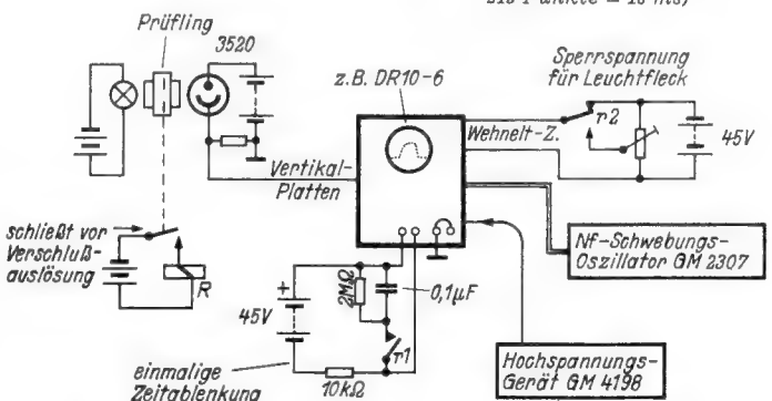
Bild 5. Anordnung zur Verschußzeitenmessung mit Lichtquelle und Fozozelle
