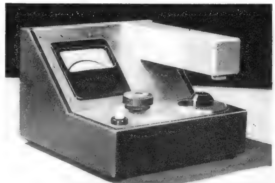
Bild 2. Absorptionsmesser zur Messung von Trübungs- und Farbwerten (Dr. Schneider, Bad Kreuznach)
