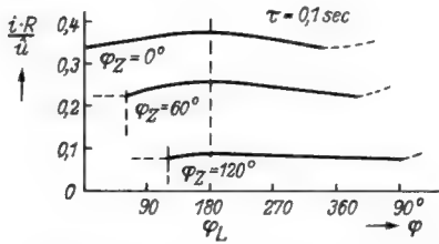
Bild 4. Stromverlauf einer Einphasenschaltung nach Bild 3 bei \tau=0,1 \text{ sec}
