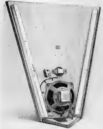
Bild 11. Celophon-Schallecke, Rückansicht einer Eckenlautsprecherkombination von Lorenz
