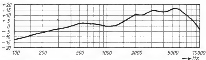
Bild 3. Frequenzkurve des Sprachmikrofons MD 7 (Labor Wennebostel)
