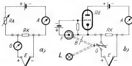
Bild 1. Kompensationschaltungen. RA = Abgleichwiderstand, RK = Kompensationswiderstand, G = Steuergalvanometer, E = Meßspannung, A = Anzeigegerät, L = Glühlampe, B = Blende 1a = Kompensationschaltung nach Lindeck-Rothe; 1b = Grundschaltung des Fotozellenkompensators von Gossen. An die Stelle des Abgleichwiderstandes RA ist die Kombination Röhre + Fotozelle getreten.
