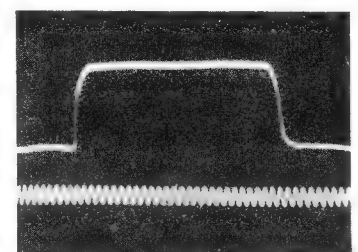
Bild 7. Verschußmessung mit Fozozelle und besonderer Eichschwingung
