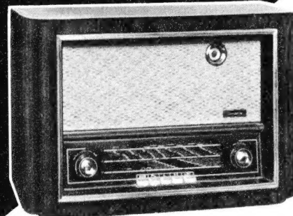
JOTHA- Mercedes 54 Großsuper mit 9 UKW- und 6 AM-Kreisen, 5 Drucktasten, 3 Wellen- bereiche, 8 Röhren, überragende UKW-Leistung durch rauscharme 2-Röhren-Hochleistungs-Vorstufe und Ratio-Detektor, großer 6-Watt-Oval-Konzert- lautsprecher, 5-Watt-Endstufe, Schwungradantrieb, Magisches Auge, geeicht. UKW-Namenskala, kontin. Tonblende, eingebauter Allwellen-Hochleistungs- Dipol, Anschlüsse für Tonabnehmer u. 2 Lautsprecher, reichverziertes, hochglanzpoliertes Edelholzgehäuse 520 x 345 x 250 mm Preis: DM 295.-
