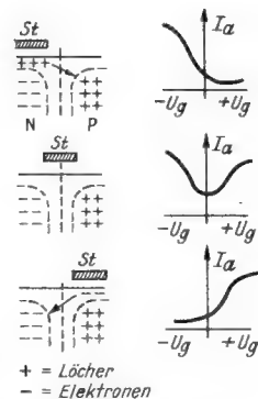
Bild 5. Einfluß der Stellung der Steuerelektrode auf den Anodenstrom eines p-n-Feldistors
