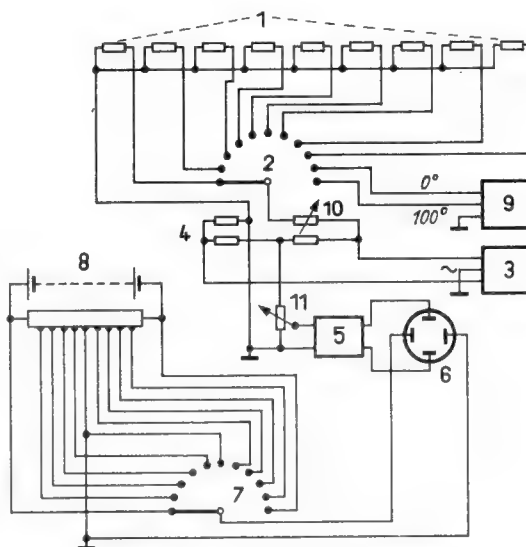
Bild 2. Prinzipschaltbild des elektronischen Thermometers (Bedeutung der Zahlen im Text)
