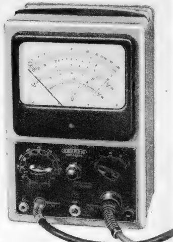
Grundig-Universal-Röhrenvoltmeter
