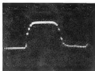
Bild 6. Verschußmessung nach Bild 5 mit Helligkeitssteuerung (Zeiteichnung mit 1,5 kHz; 18 Punkte = 12 ms, davon 12 Punkte = 8 ms volle Öffnung)
