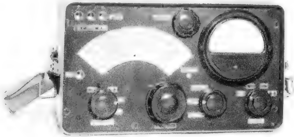
Bild 7. Kathrein-Antennen-Testgerät
