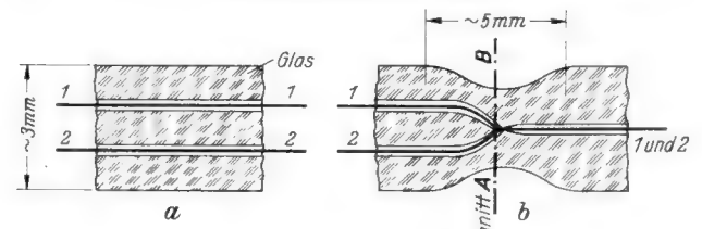
Bild 2. Herstellung des geringen Elektroden-Abstandes durch Einschmelzen von Drähten in einen Glasstab
