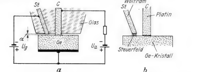
Bild 1. Punktkontakt-Fieldistor. a = grundsätzliche Schaltung, b = Anordnung der Elektroden
