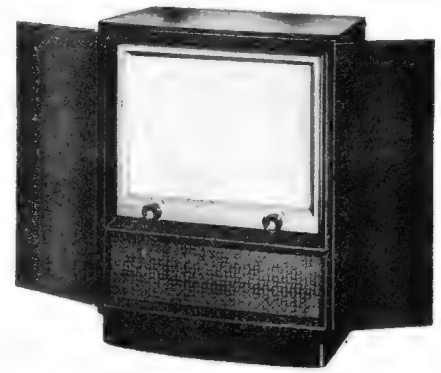
Bild 6. Grundig-Fernsehschrank 710 mit „Magischem Rahmen“ (erleuchteter Bildfeldumrandung)
