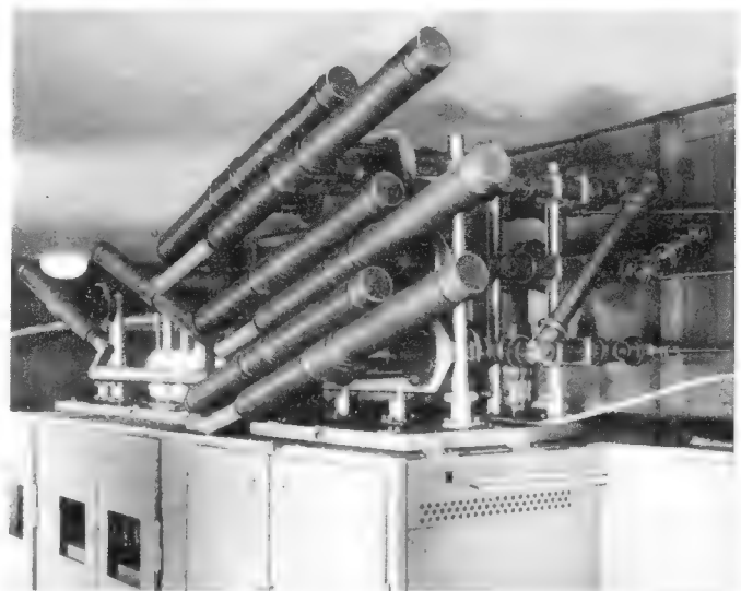
Kein Raketenwerfer, sondern das Einseitenbandfilter des neuen Lorenz-Fernsehenders auf dem großen Feldberg. Es unterdrückt, wie der Name andeutet, das eine Modulations-Seitenband der Bildsenderfrequenz. Eine weitere Einrichtung, der Diplexer (links im Hintergrund), entkoppelt Bild- und Tonsender, so daß sie gemeinsam an eine Antenne angeschlossen werden können. Beide Einrichtungen sind in einer neuartigen Technik als „Brücken“ in Form koaxialer Ringleitungen ausgeführt
