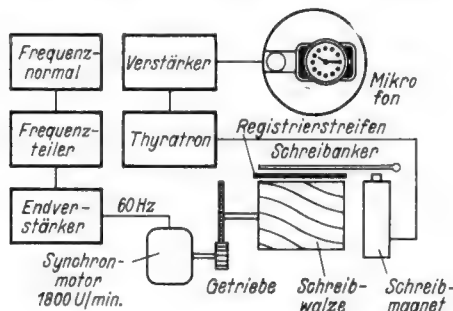
Bild 1. Prinzipschaltbild der Zeitwaage. Das Frequenznormal bestimmt die Drehzahl des Synchronmotors und damit Geschwindigkeit des Registrierstreifens und Drehzahl der Schreibspiralen. Die Laufgeräusche der zu prüfenden Uhr betätigen über das Thyatron den Anker des Schreibmagneten. Röhrenaufwand: 9 Röhren
